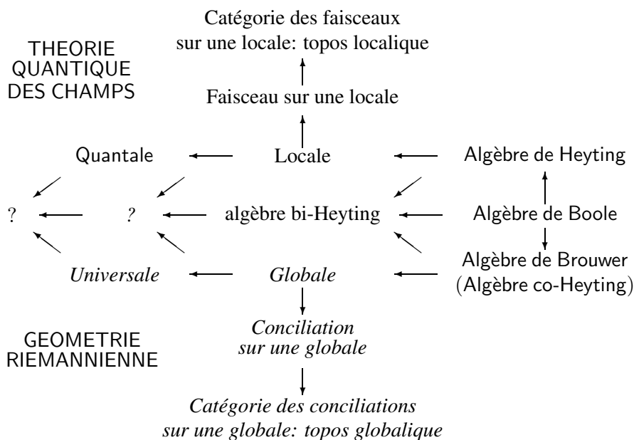
Le diagramme de Majid complété et M-dualisé
